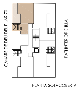
PLANTA SOTACOBERTA
